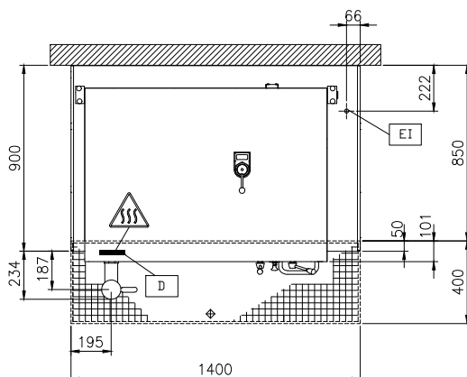
Boven aanzicht
